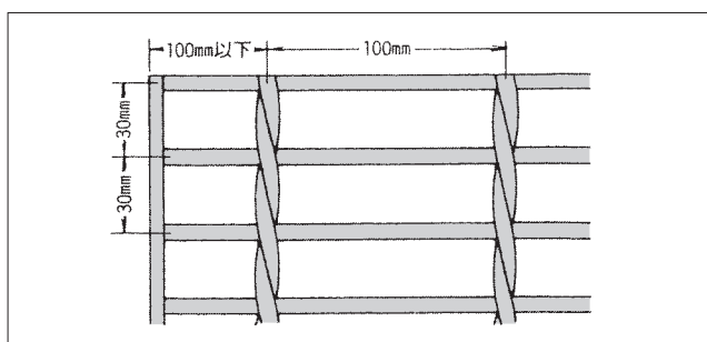
●クローズエンド式 両端部にベアリングバーと同じ高さのフラットバー（エンドバーと云う）をあてて縁取りをしたものです。
