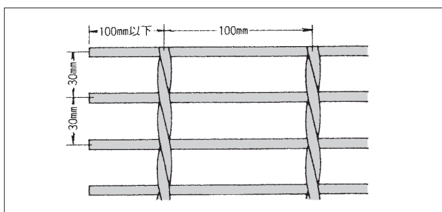
●オープンエンド式 両端部が切りっぱなしのもの
