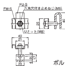
〈H19~H44〉
