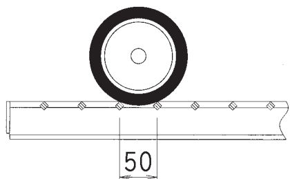
■クロスバーピッチ 50mm
