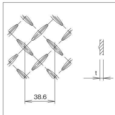
縞目の寸法 板厚は3.2mm/4.5mm/6.0mmです。
