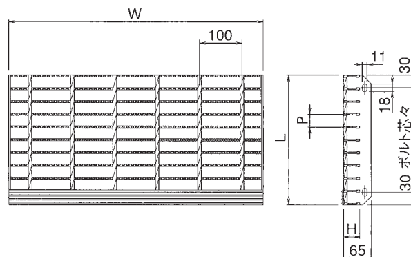
ボルト式
