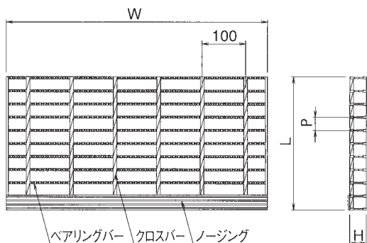
溶接式
