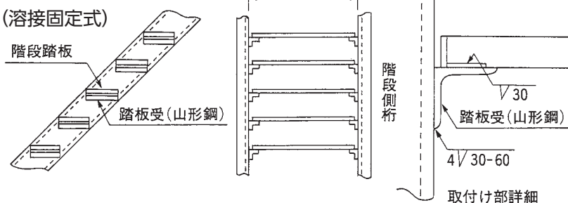
(B) 階段踏板取付け方法(ボルト固定式)
