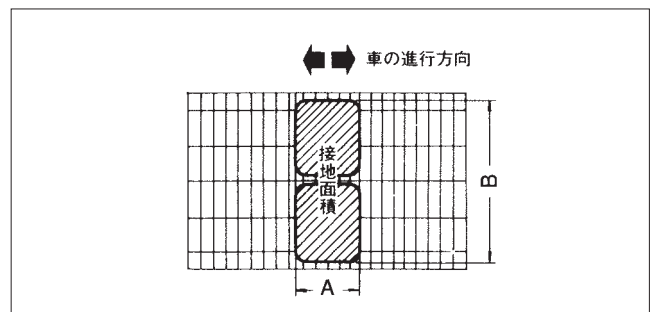
側溝の場合
