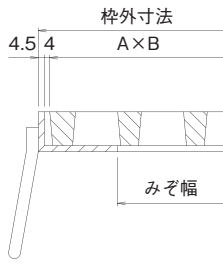
受枠との納まり図
