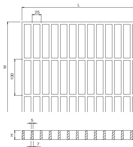
■寸法表 (CYBZ-N5)
