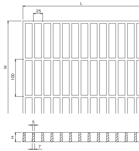
■寸法表 (CYBZ-N5) (単位: mm)
