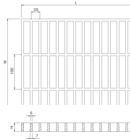
■寸法表 (CYBZ-N5)
