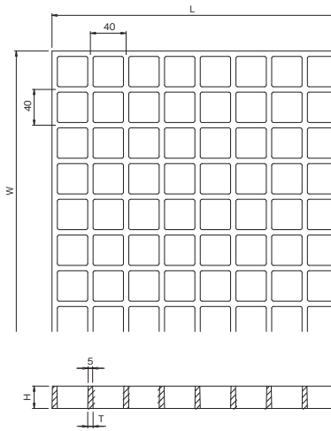
■寸法表 (CYBZ-N10) (単位: mm)
